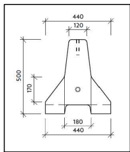
BETONOVÉ SVODIDLO 2000/440/500 MM
